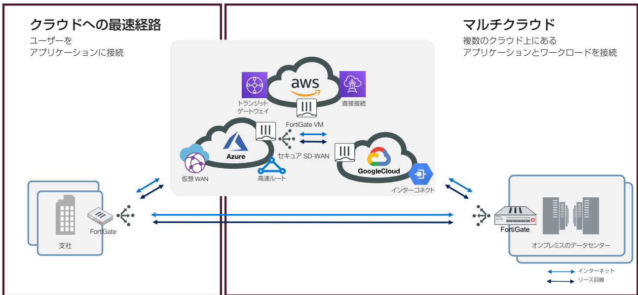
図 2：フォーティネットのクラウド向けセキュア SD-WAN。ユーザー、アプリケーション、クラウド接続のユースケース。
